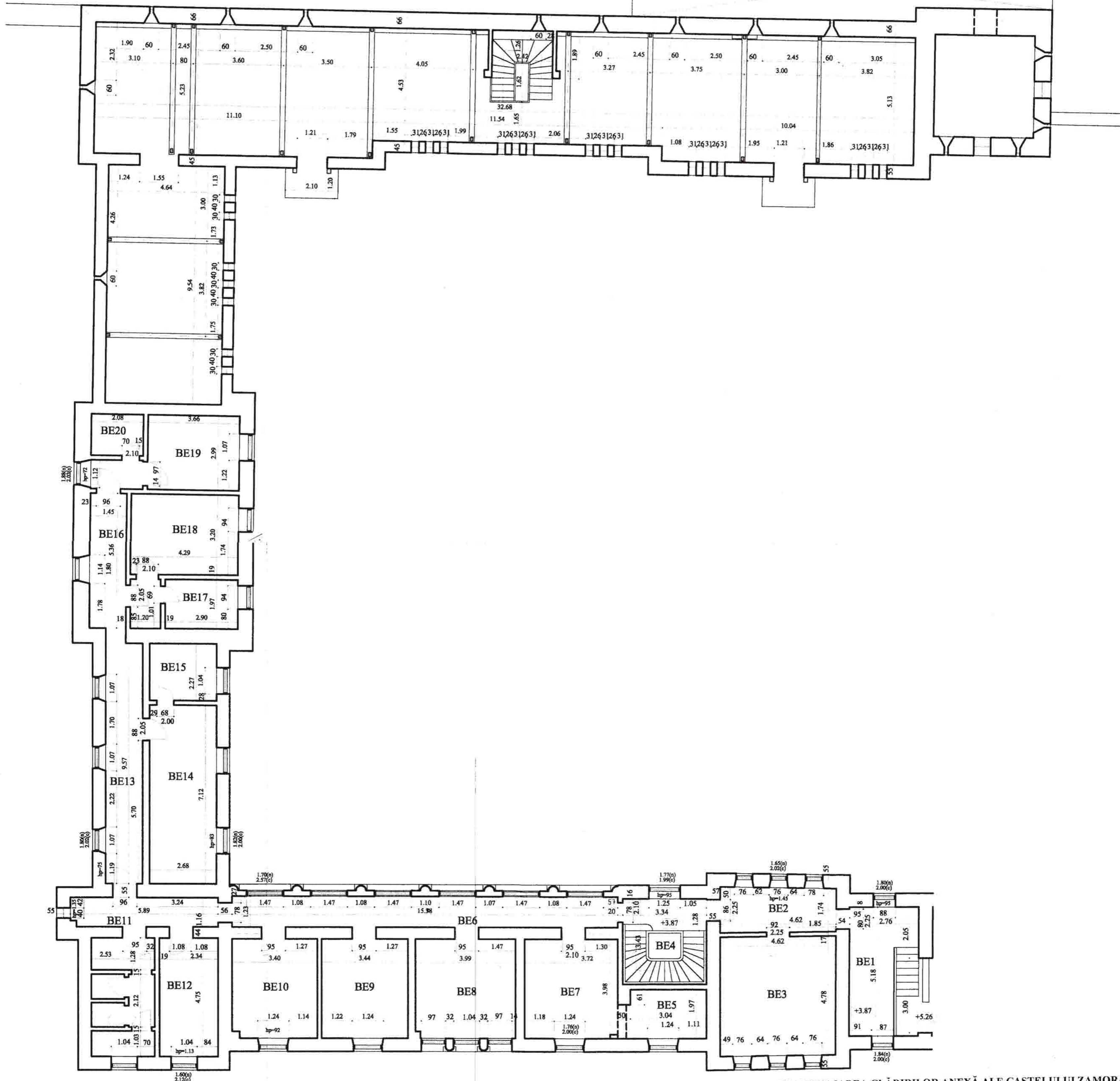
PLAN ETAJ cota +3.87 sc. 1:100 RELEVU
